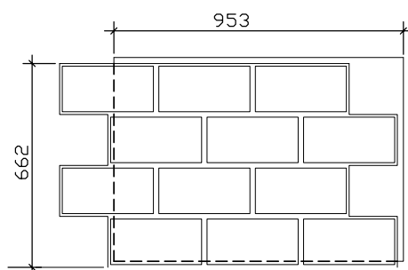
Рис. 9. Термопанель ППУ цокольная
