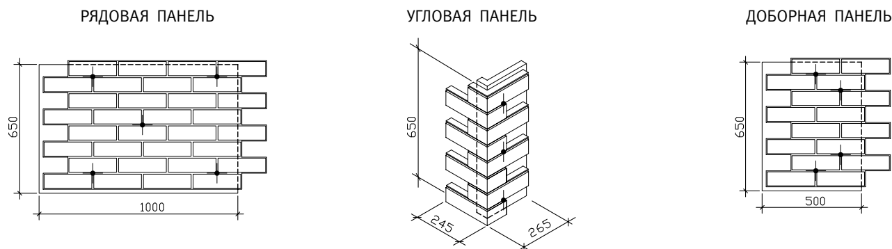
Рис. 4. Термопанель ППС по технологии полимерного соединения
