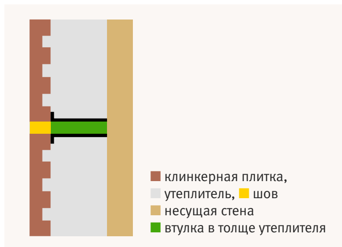
Рис. 18.1 Крепление термопанели на основе ППС
