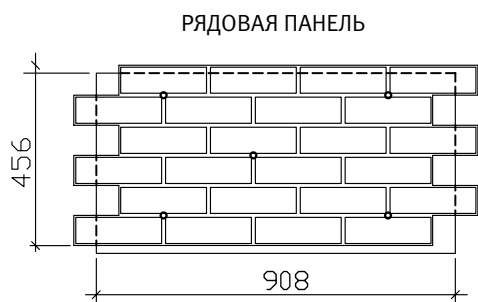
Термопанель рядовая на основе экструдированного пенополистирола с облицовочной плиткой формата 217х66 мм
