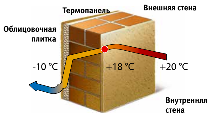
Рис. 19.2. Стена с утеплителем. Значительное снижение теплопотерь через утеплённую стену с внешней стороны вызывает повышение температуры её внутренней поверхности
