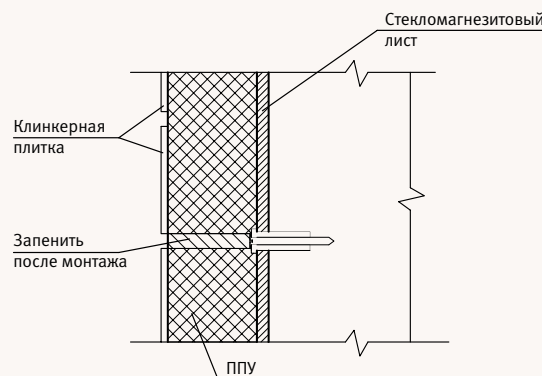
Рис. 18.2 Узел крепления термопанели на основе ППУ
