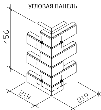
Термопанель угловая на основе экструдированного пенополистирола с облицовочной плиткой формата 217х66 мм
