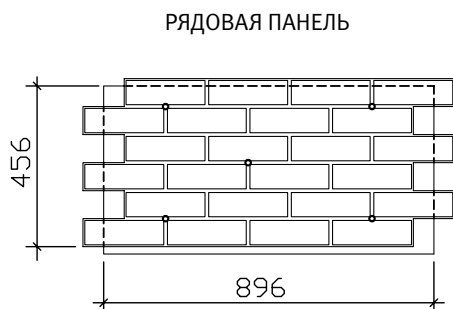
Термопанель рядовая на основе экструдированного пенополистирола с облицовочной плиткой формата 214х66 мм
