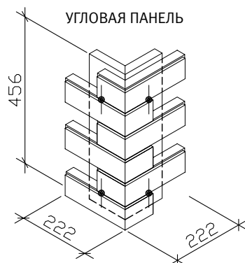
Термопанель угловая на основе экструдированного пенополистирола с облицовочной плиткой формата 217х66 мм
