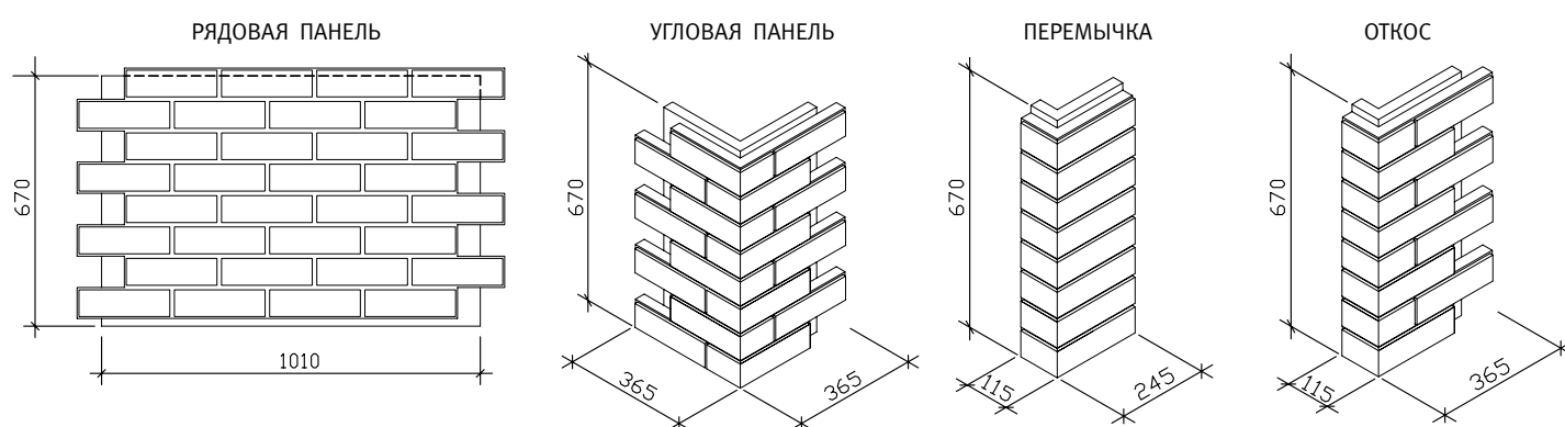
Рис. 8. Термопанель ППУ
