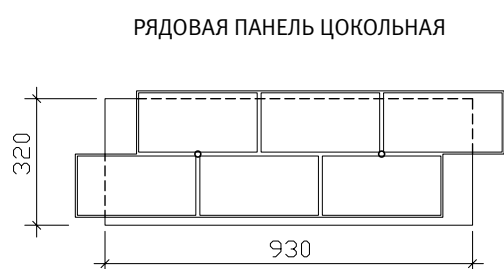
Термопанель рядовая цокольная на основе экструдированного пенополистирола с облицовочной плиткой формата 300х150 мм
