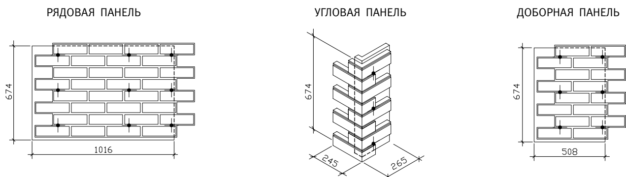
Рис. 7. Термопанель ППС по технологии термопрессования клинкерной плитки
