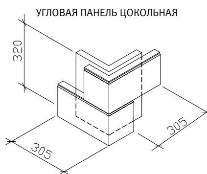
Термопанель угловая на основе экструдированного пенополистирола с облицовочной плиткой формата 214х66 мм
